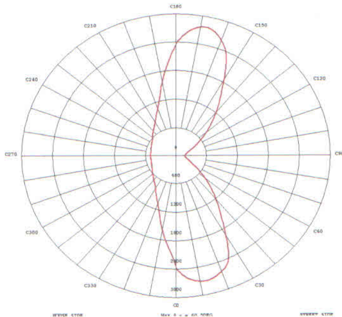
Figura 2 - Curva de intensidade máxima para cada ângulo C
