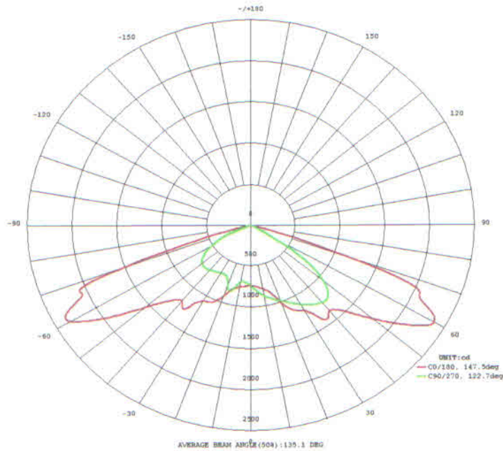
Figura 1 - Curva de distribuição de intensidade luminosa
