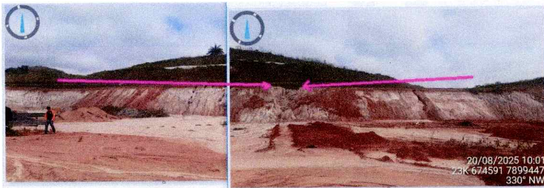
Imagem 02: Falha construtiva da berma que proporciona acúmulo de água na crista do talude e desencadeia processos erosivos.
