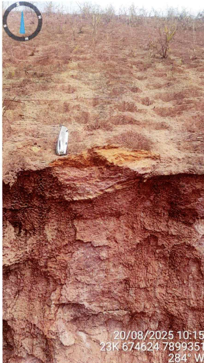
Imagem 12: Detalhe do contato do material mais frível sotoposto ao material mais competente
